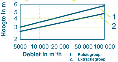
Afmetingen van luchtgroepenlokaal
