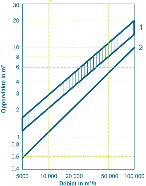
Afmetingen van technische kokers
