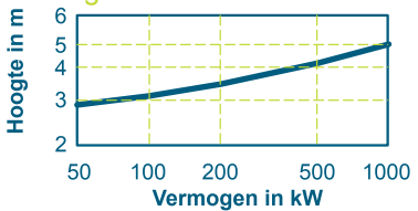
Afmetingen van koeltechnisch lokaal
